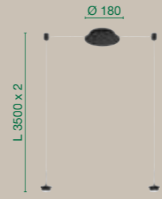
3804-42-101 16W - 1500 lm
