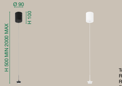
3804-45-101 8W - 750 lm
