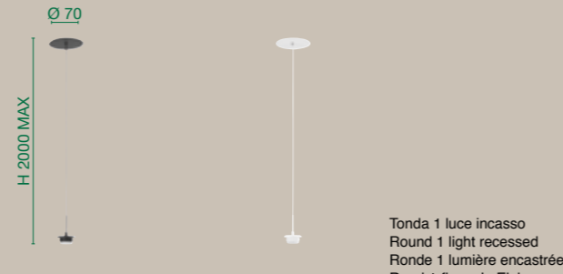
3804-40-101 8W - 750 lm
