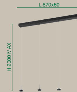
3804-48-101 28W - 3000 lm
