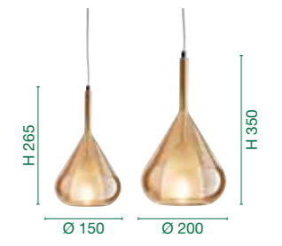
3481-59-125 3481-50-125 E14 40W E27 40W
